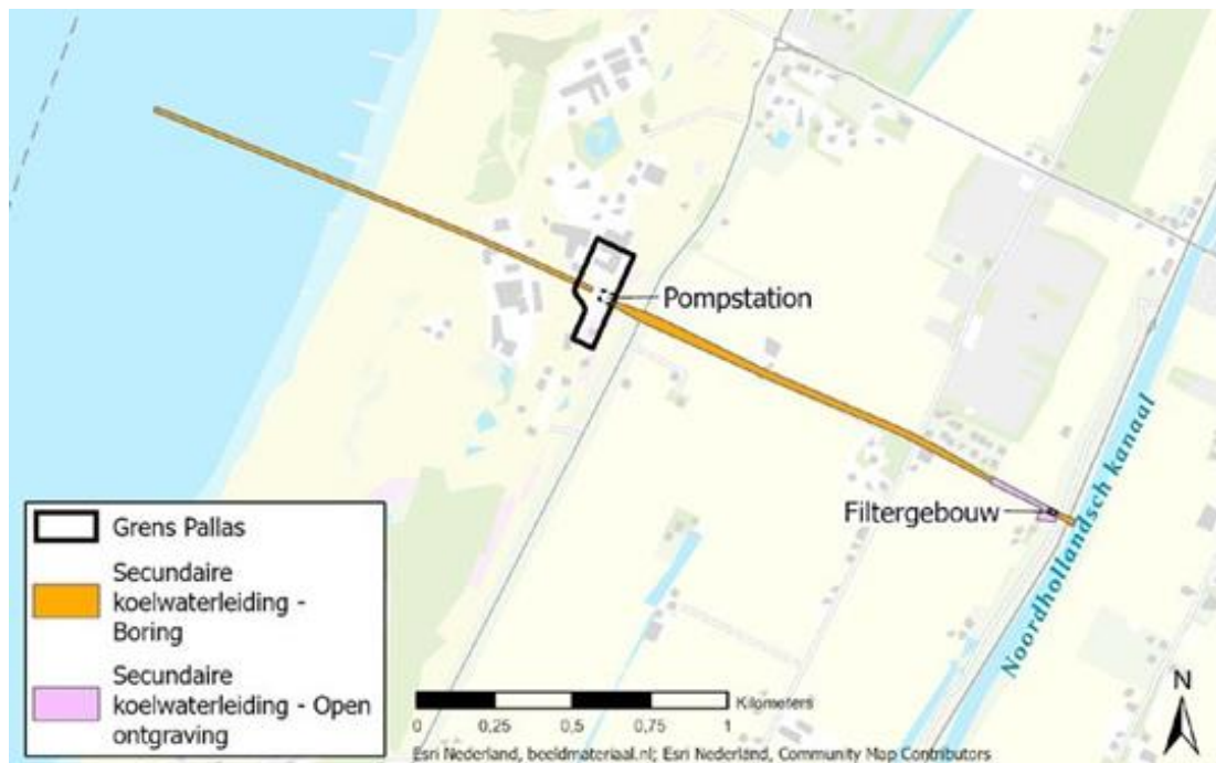
Figuur 7 Tracé van de koelwaterleiding (van filtergebouw (Canal Intake Building) via pompstation (SCS-building met surgetower) naar de Noordzee) ten behoeve van de PALLAS-reactor. Aan het oostelijke uiteinde bevindt zich het onttrekkingspunt in het Noordhollandsch Kanaal, aan het westelijke uiteinde (circa 650 m uit de Rijkstrandpalenlijn) het lozingspunt in de Noordzee.
